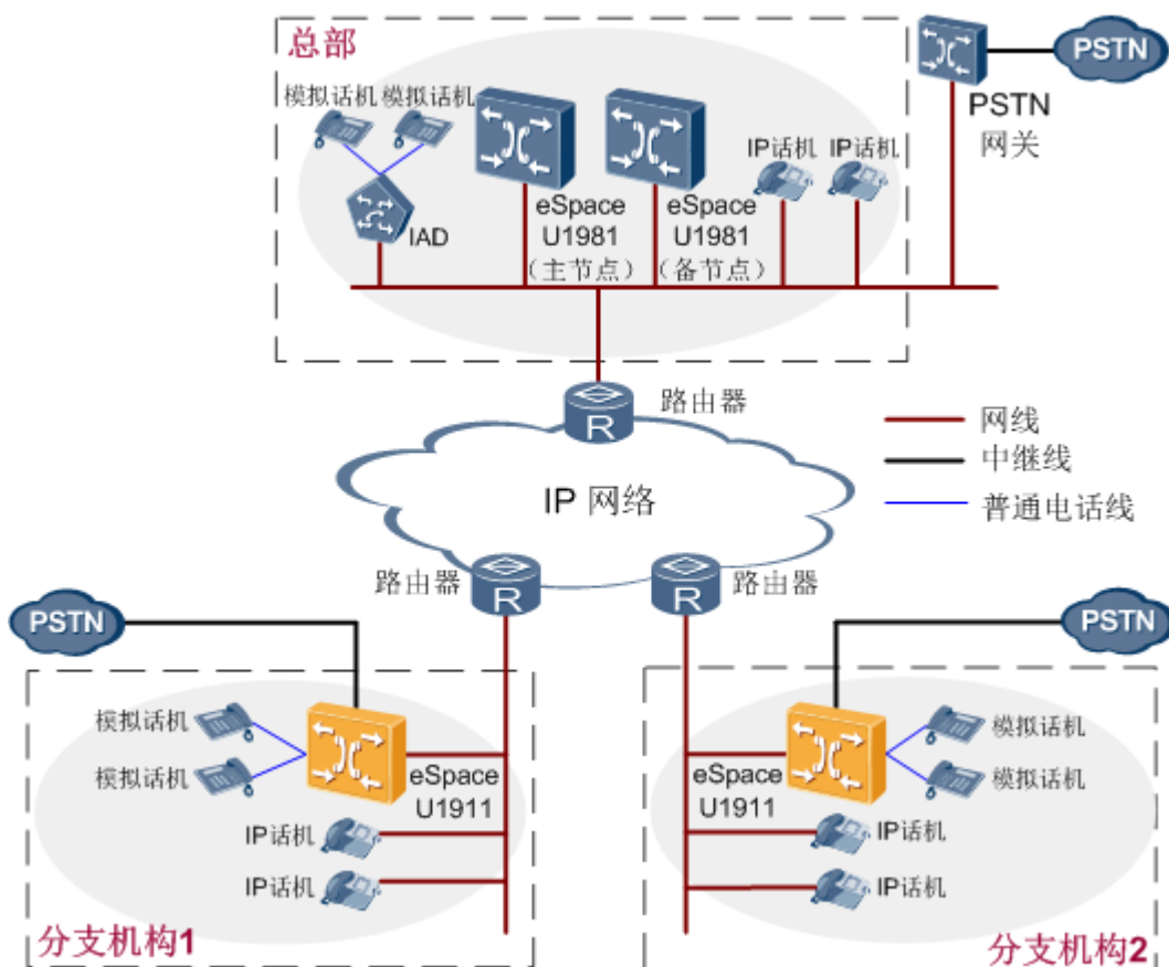
图 2-2 分布式组网
