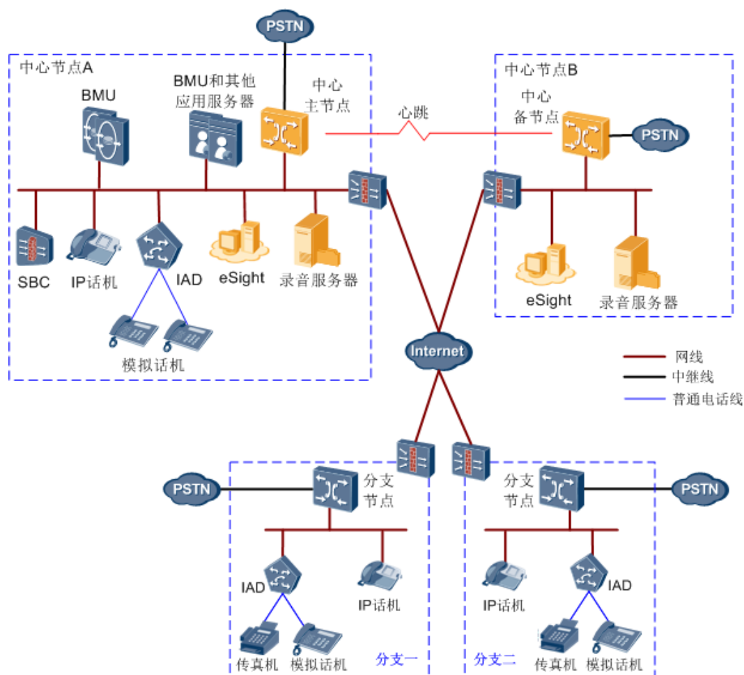
图 2-3 异地容灾典型组网
