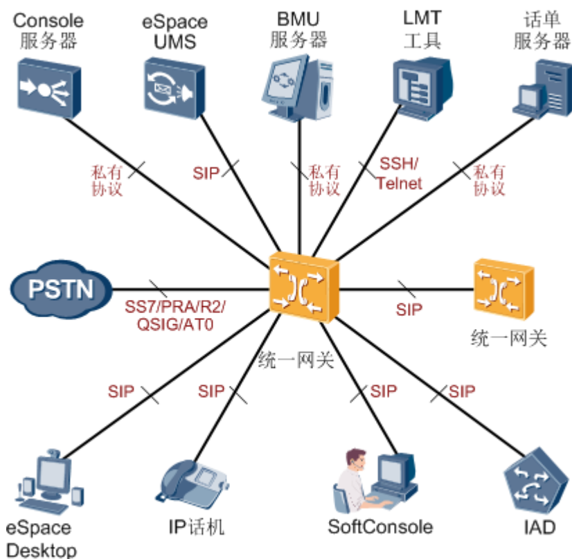
图 6-1 对外接口的信令协议分布
