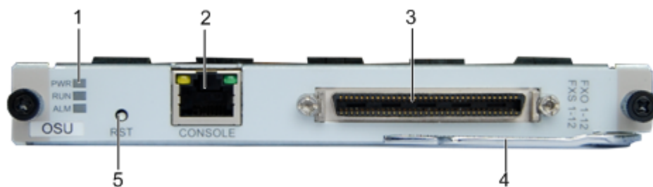
图 3-9 OSU 面板外观
