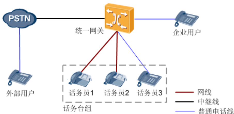
图 4-1 硬话务台组网
