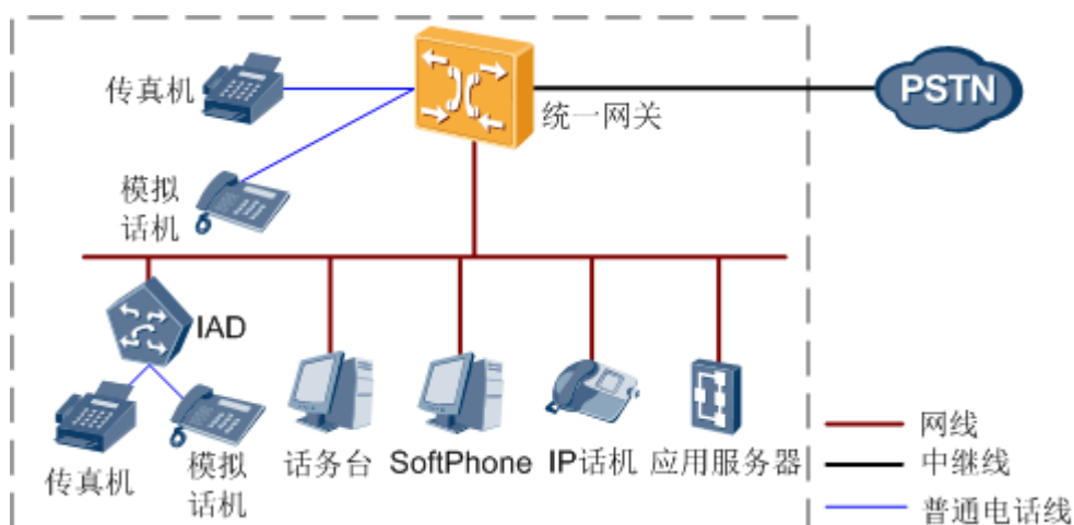
图 2-1 集中式组网
