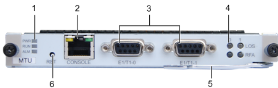
图 3-5 MTU 面板外观
