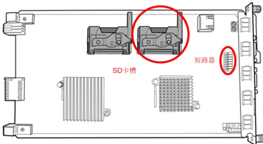
图 3-6 重要器件位置
