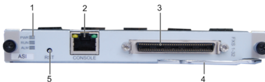
图 3-8 ASI 面板外观
