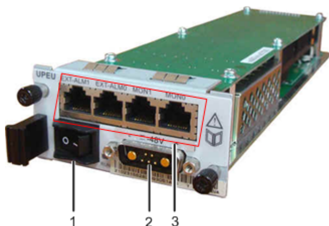
图 3-11 直流电源模块外观
