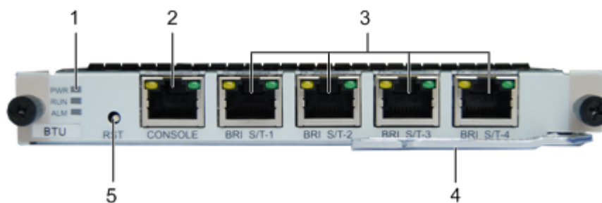
图 3-7 BTU 面板外观
